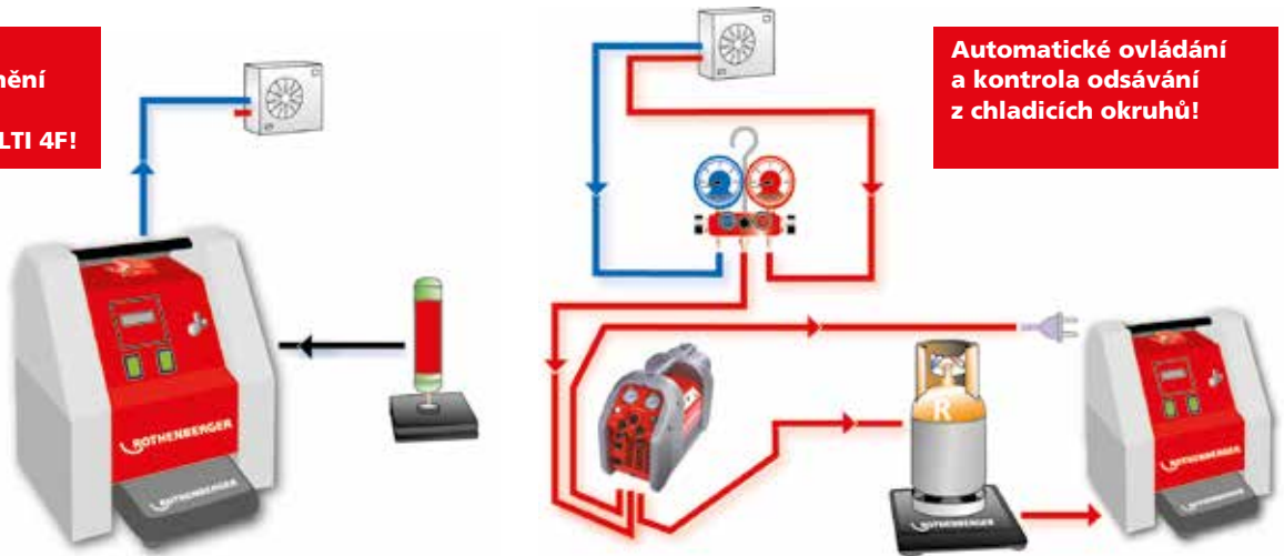
ROKLIMA® MULTI 4F při použití (evakuace & plnění)
